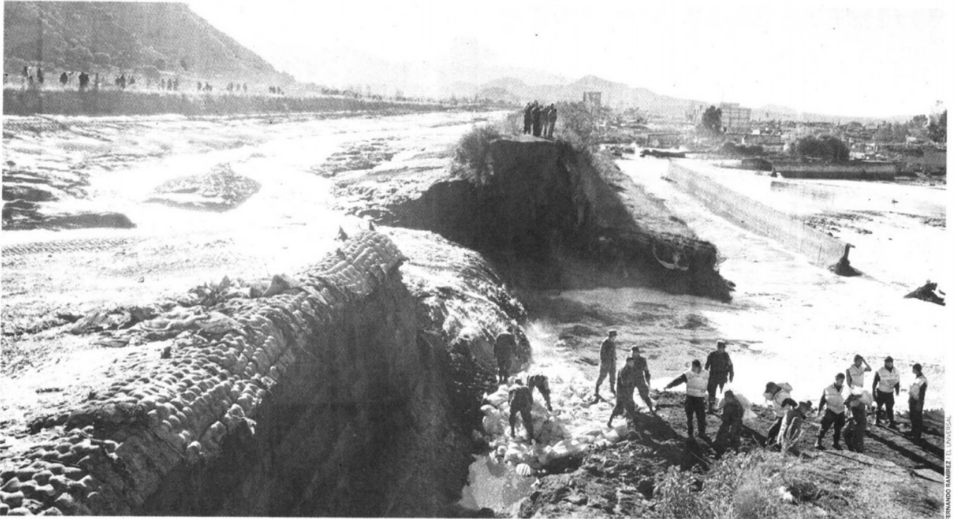
FUGA. Por la fractura de 50 metros del canal de La Compañía se desparrramaban 50 litros por segundo hacia las comunidades chalquenses; la prioridad era sellar el escape y luego rebombear las aguas residuales
